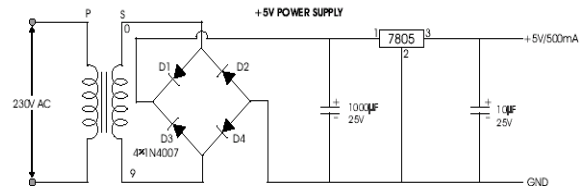
Fig-5:bridge rectifier
